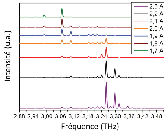
FIGURE 5.12 – Spectres d'émission pour différentes valeurs de courant I_{th} < I < I_{max} à basse température ( T = 78 K).
