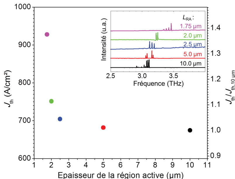
FIGURE 5.15 – Densité de courant de seuil ( J_{th} ) en fonction de l'épaisseur de la région active ( L_{RA} ) à basse température ( T = 10 K). Encart : Spectres d'émission au seuil laser pour les cinq épaisseurs à T = 10 K.
