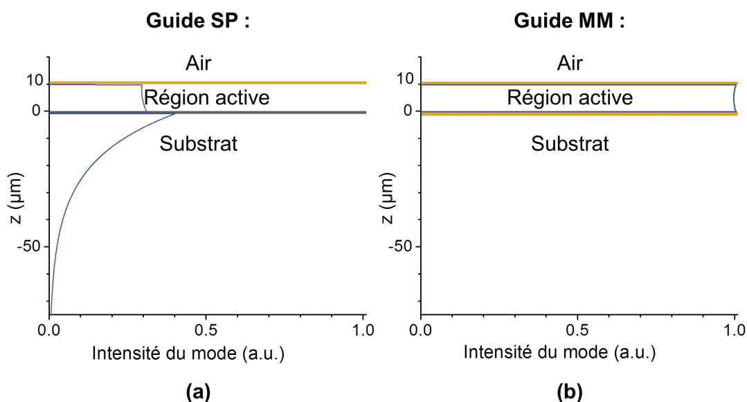
FIGURE 4.4 – Amplitude de la composante principale du champ électrique ( E_z ) pour le mode \text{TM}_0 selon la direction de confinement ( z ) : comparaison entre un guide SP (a) et un guide MM (b) d'épaisseur L_{\text{RA}} = 10 \mu\text{m} , pour \lambda = 100 \mu\text{m} . En jaune : couche mince métallique. En gris : couche mince de GaAs dopé n+.
