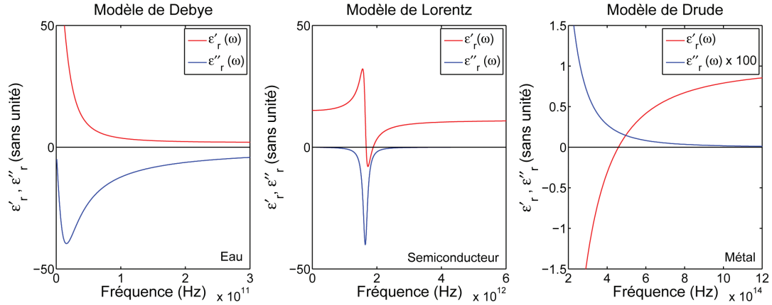
FIGURE 1.8 – A gauche : Modèle de Debye. Partie réelle (courbe rouge) et partie imaginaire (courbe bleu) de la fonction de permittivité diélectrique de l'eau calculée par la méthode de Debye, avec \epsilon(0) = 81 , \epsilon_\infty = 1.8 et \tau_d = 10 ps, en fonction de la fréquence. Au milieu : Modèle de Lorentz. Partie réelle (courbe rouge) et partie imaginaire (courbe bleu) de la fonction de permittivité diélectrique d'un matériau semiconducteur calculée par la méthode de Lorentz, avec N = 1e^{15} \text{ cm}^{-3} , \epsilon_\infty = 11 , \omega_0 = \frac{\omega_p}{2} et \gamma = \frac{\omega_0}{10} , en fonction de la fréquence. A droite : Modèle de Drude. Partie réelle (courbe rouge) et partie imaginaire (courbe bleu) de la fonction de permittivité diélectrique d'un matériau métallique calculée par la méthode de Drude, avec \epsilon_\infty = 1 , \hbar\omega_p = 1.9 eV et \tau_d = 30 fs, en fonction de la fréquence.
