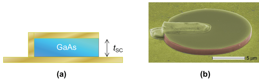
FIGURE 3.3 – Schéma (a) et image SEM (b) d'un résonateur hybride fabriqué à partir d'un micro-disque "patch".
