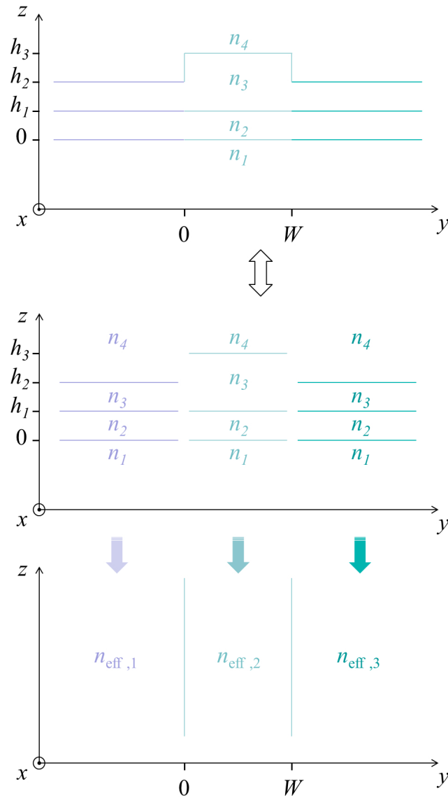
FIGURE 1.7 – Méthode de l'indice effectif : exemple d'un guide d'onde 2D composé à partir de quatre matériaux d'indices n_i , que l'on peut diviser en trois guides d'ondes indépendants 1D dont on peut calculer les indices effectifs n_{\text{eff},j}
