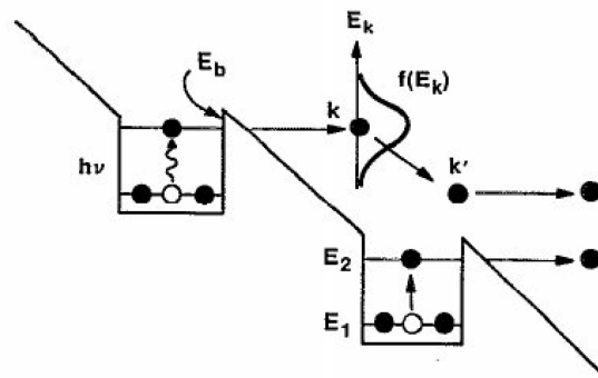
FIGURE 4 – Principe général d'un QWIP [87].
